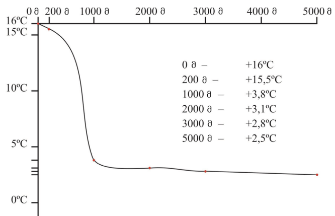
ოკეანეებში ტემპერატურის ცვლილების სიღრმეზე დამოკიდებულება
