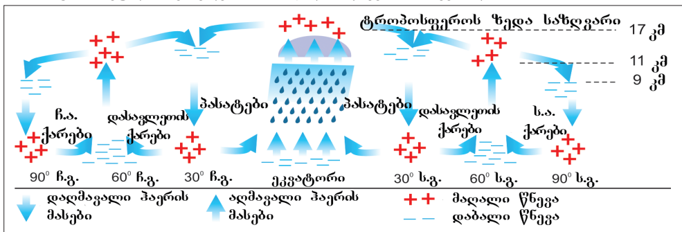
ტროპოსფეროში ჰაერის ბრუნვის ზოგადი სქემა
