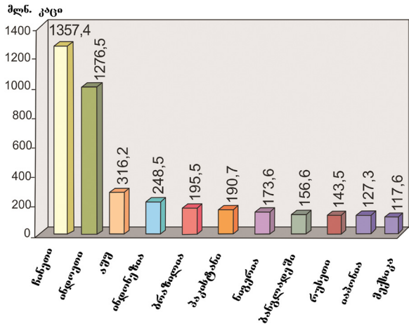
მოწინავე ქვეყნები, მოსახლეობის რაოდენობის მიხედვით (2013)
