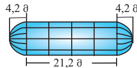
თხევადი წყალბადის ავზი
