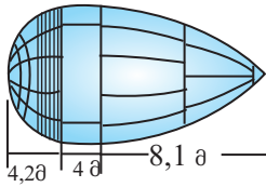
თხევადი ჟანგბადის ავზი
