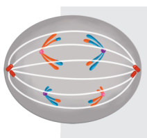
Анафаза I
