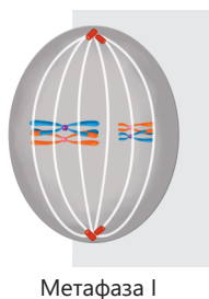
Метафаза I
