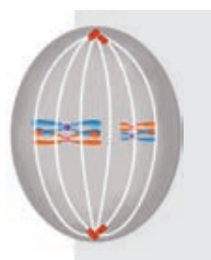
Метафаза I
