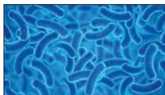
Молочнокислые бактерии
