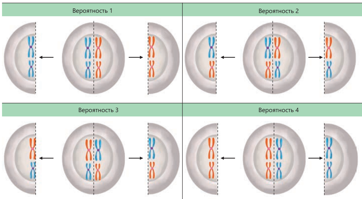
Метафаза I
