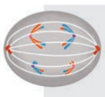
Анафаза I
