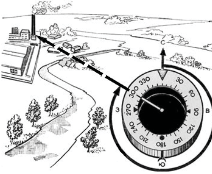
Adrianov kompası ilə maqnit azimutunun təyini. Şəkində zavod borusuna olan istiqamətin maqnit azimutu 300°-dir.
