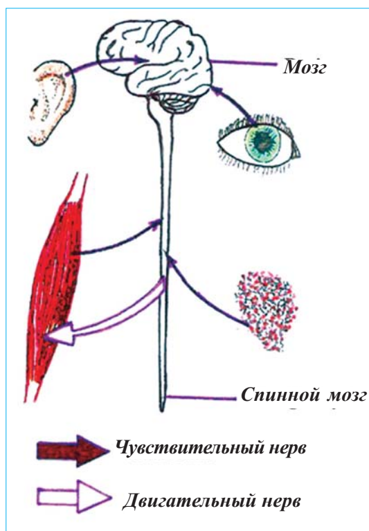
Рис 7. Рефлекторная дуга
