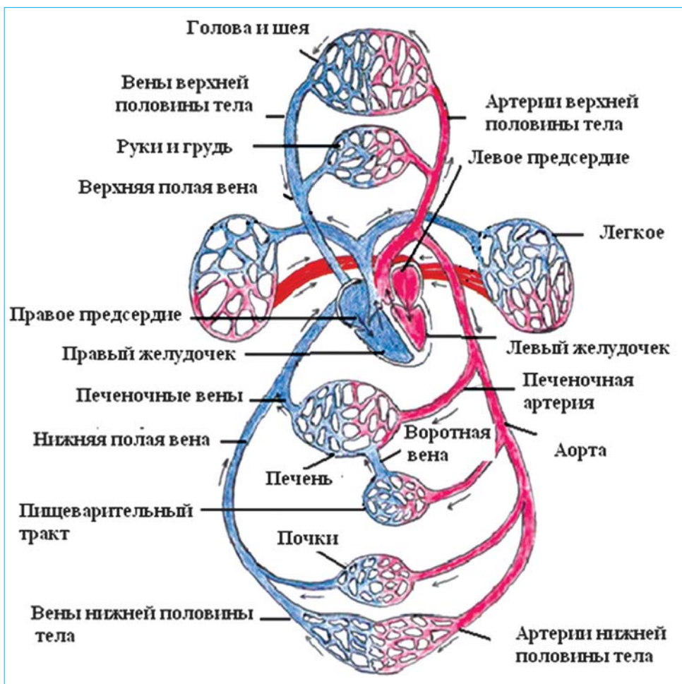
Рис 6. Схема кровообращения
