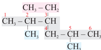
2,5-диметил-3-этилгексан
