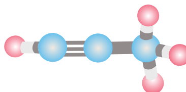
шаростержневая модель молекулы пропина
