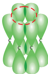
Образование общей \pi - системы в молекуле бензол
