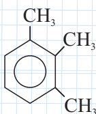
1,2,3-триметилбензол
