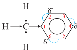
Перемещение электронной плотности в молекуле толуола
