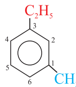
1-метил-3-этилбензол
