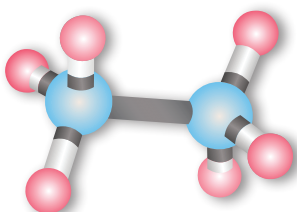
Шаростержневая модель молекулы этана
