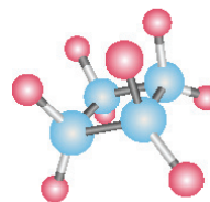
шаростержневая модель молекулы циклобутана
