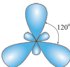
Форма sp^2 - гибридных
