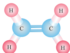
Шаростержневая модель молекулы этена
