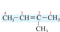
2-метилбутан-2
