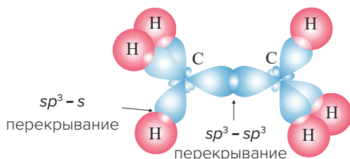
Схема образования \sigma -связей в молекуле этана
