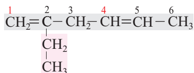
2-этилгексадиен-1,4
