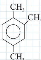
1,2,4-триметилбензол
