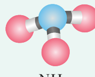
NH_3
