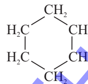
циклогексан
