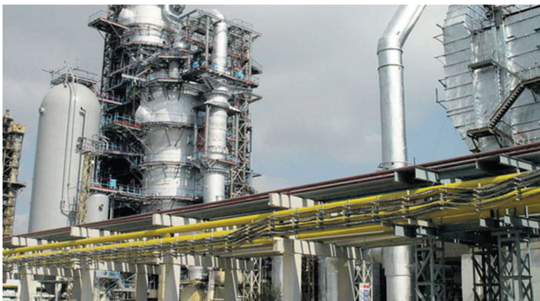
Крекинговое оборудование Бакинского нефтеперерабатывающего завода
