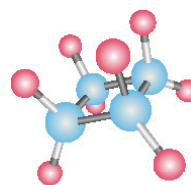
tsiklobutan molekulunun mil-kürəcik modeli
