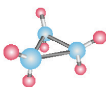
tsiklopropan molekulunun mil-kürəcik modeli
