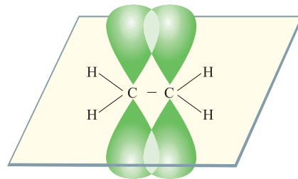
Eten molekulunda \pi -rabitənin əmələgəlmə sxemi
