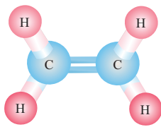
Eten molekulunun mil-kürəcik modeli
