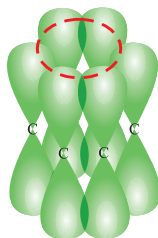
Benzol molekulunda ümumi \pi -sistem
