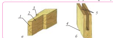
Рис. 2. Основные элементы шипа и проушины: а – шип: 1 – торец шипа; 2 – запечник; 3 – боковая грань; б – проушина: 4 – дно проушины; 5 – щечки
