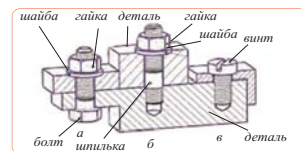
Рис. 2. Виды резьбовых соединений: а – болтовое; б – шпильное; в – винтовое
