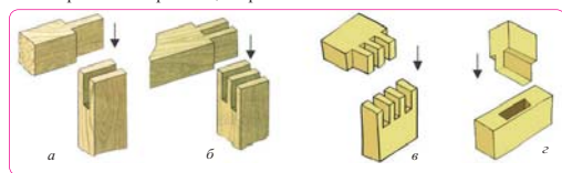
Рис. 3. Виды шиповых соединений: а – открытое одианное, б – открытое двойное, в – открытое тройное, г – прямое закрытое
