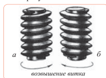
Рис. 4. Виды резьбы по направлению витка: а – правая резьба; б – левая резьба
