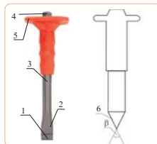
Рис. 1. Зубило
