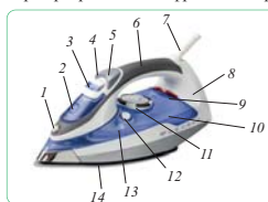
Рис. 1. Электрический утюг: 1 – разбрызгиватель воды; 2 – крышка, закрывающая отверстие для залива воды; 3 – рычажок, регулирующий постоянную подачу пара; 4 – кнопка для разбрызгивания пара; 5 – кнопка для дополнительной подачи пара; 6 – ручка утюга; 7 – вставка для защиты электрического шнура от перегибов; 8 – основа утюга; 9 – сигнальная лампочка; 10 – емкость для воды; 11 – ручка регулятора температуры глажки; 12 – включение режима самоочистки; 13 – отметка, показывающая уровень воды в резервуаре; 14 – подошва утюга
