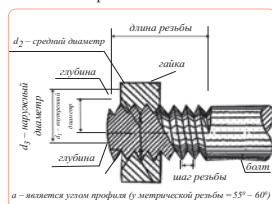
Рис. 5. Основные элементы резьбы
